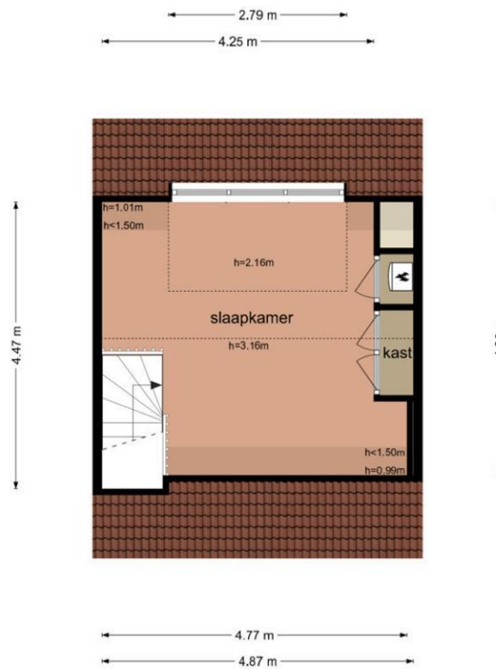
Wethouder In 't Veldstraat 66 - Amsterdam Tweede Verdieping
